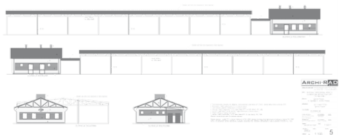
Sch. Archiwum Schemat budowy targowiska wraz z elementami infrastruktury technicznej.
